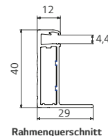
Rahmenquerschnitt
